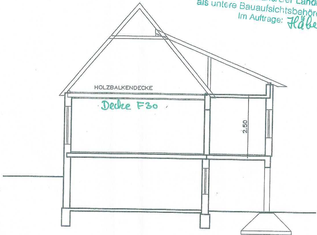
SCHNITT
