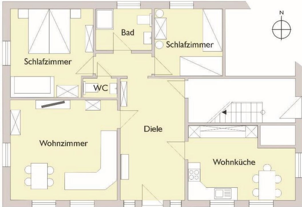
Grundriss Erdgeschoss
