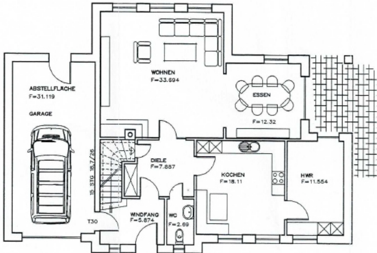
Grundriss Erdgeschoss
