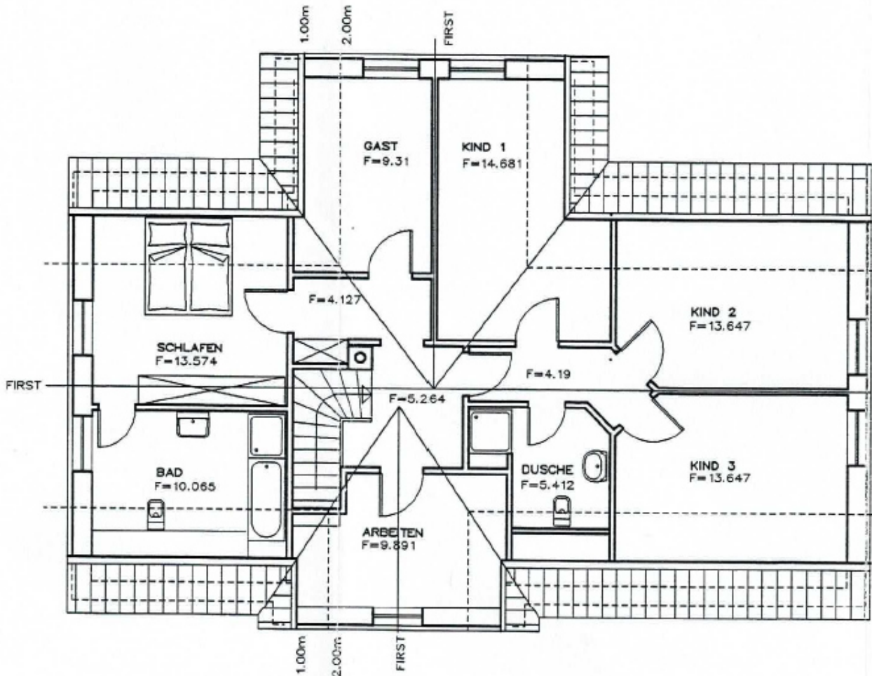
Grundriss Dachgeschoss
