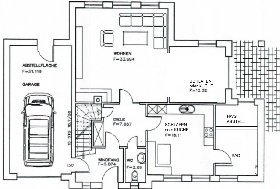
Möglicher Grundriss Wohnung 1 (EG)
