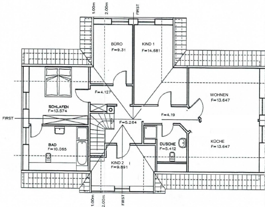
Möglicher Grundriss Wohnung 2 (DG)
